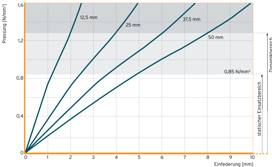
Abb. 1: Quasistatische Federkennlinie mit einer Belastungsgeschwindigkeit von 0,085 N/mm 2 /s
